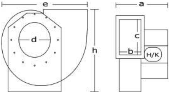
Φ300-2.0HP-1450RPM
