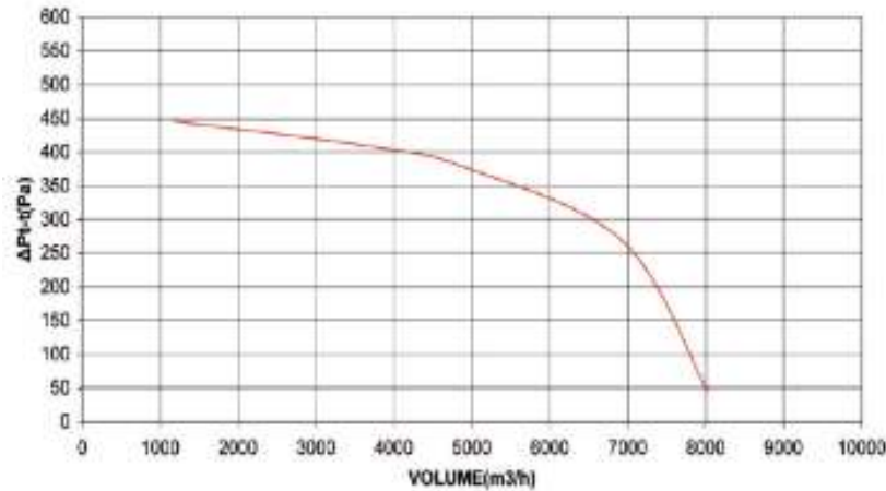
Φ300-2.0HP-1450RPM
